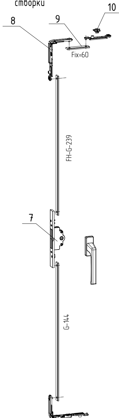
Детали фурнитуры для складной створки
