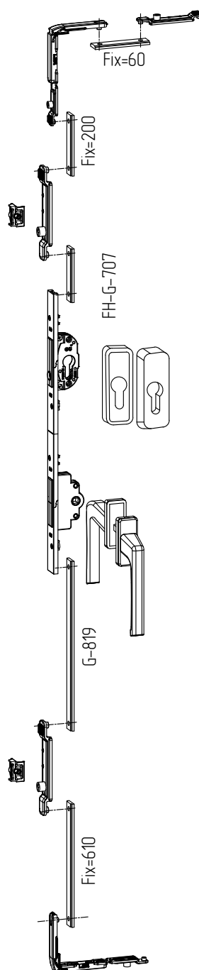
Детали фурнитуры для поворотной активной створки
